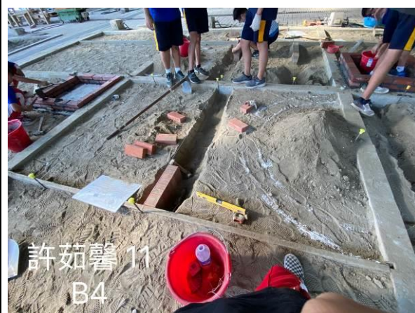
紅磚路緣施作及土丘堆置練習
