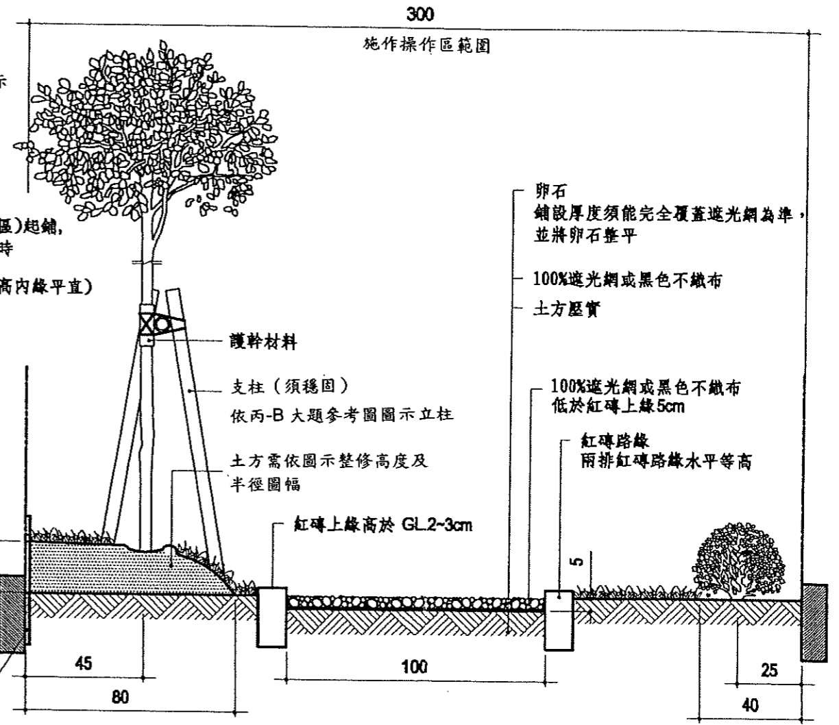
剖面圖 (A) S=1/20
