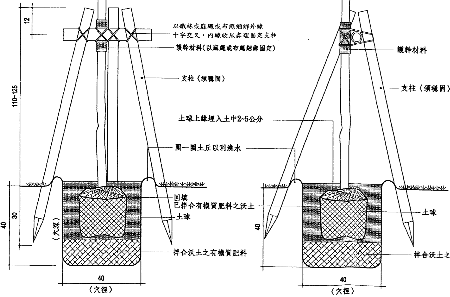
喬木栽植剖面示意圖 S=1/10
