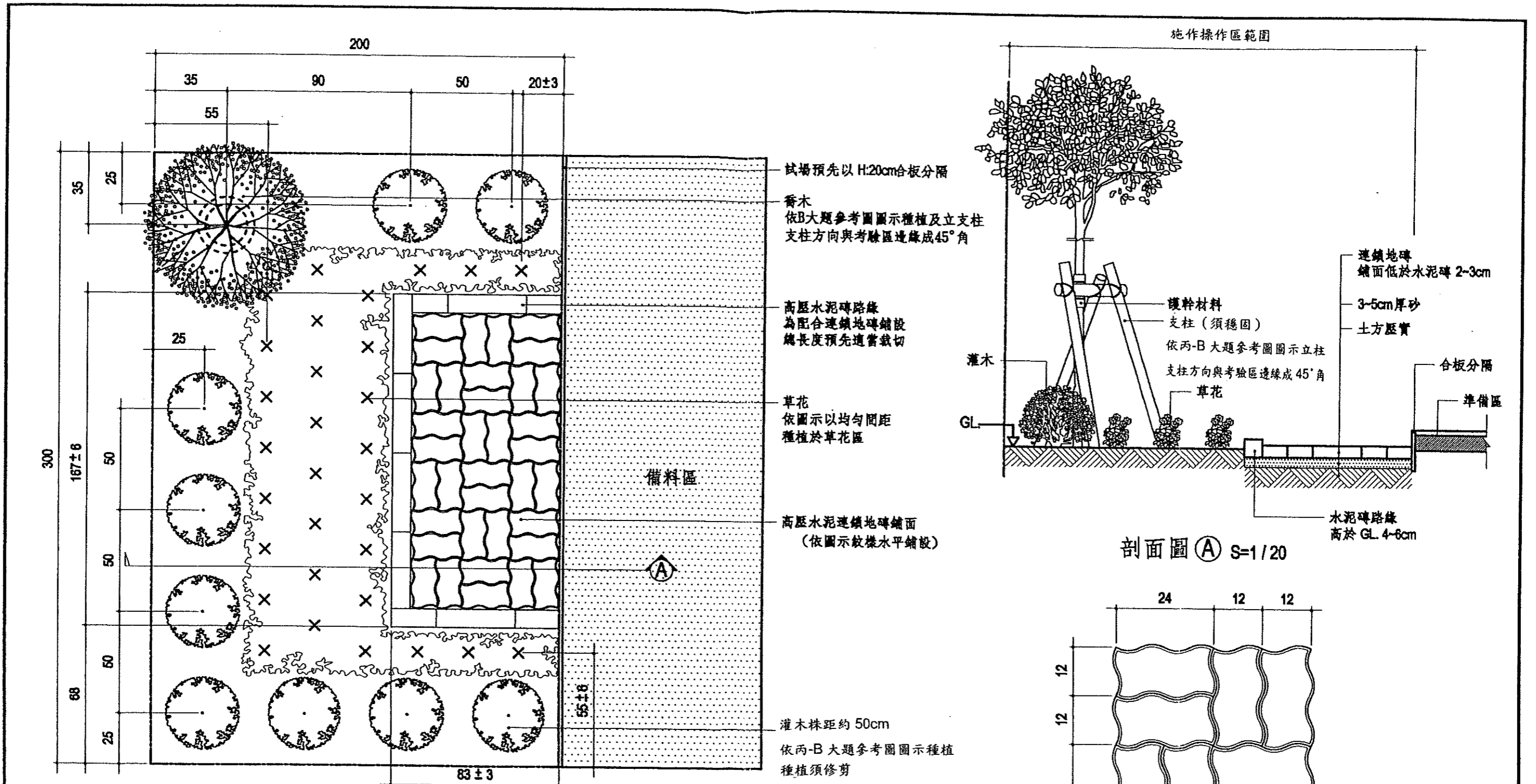
平面圖 S=1/20
