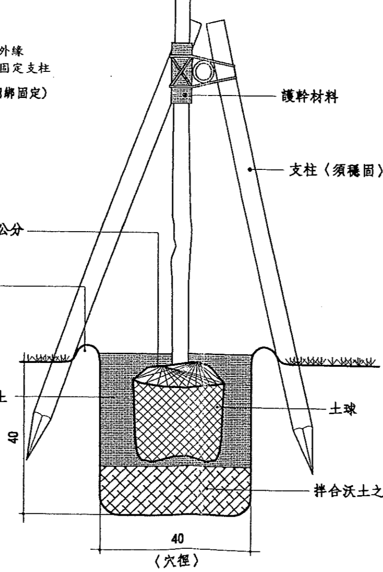
喬木栽植剖面示意圖〈側面〉S=1/10
