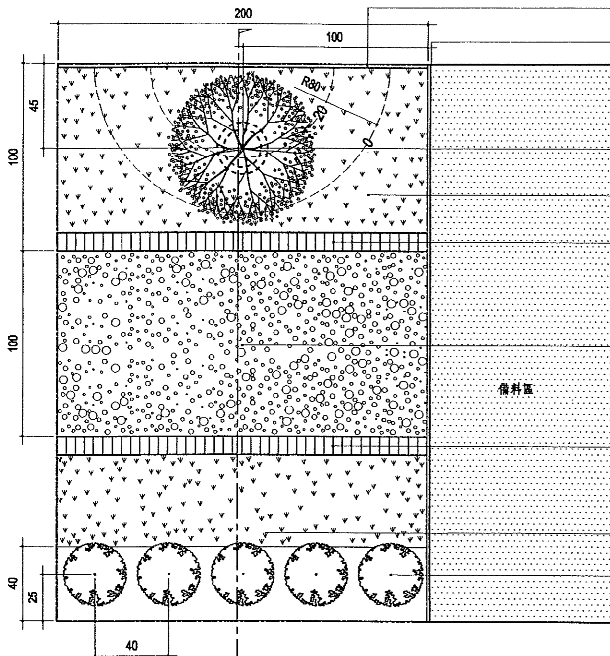
平面圖 S=1/20
