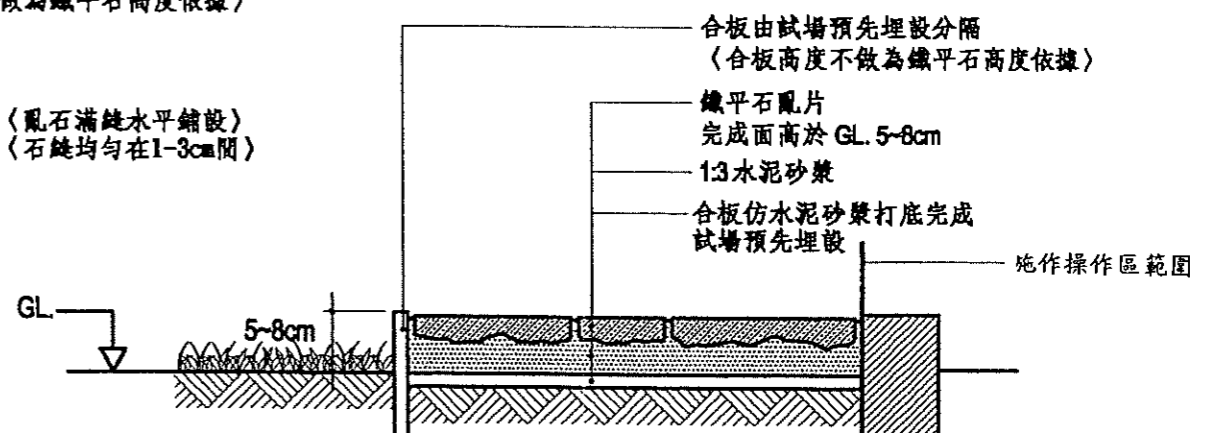
剖面圖 B S=1/10
