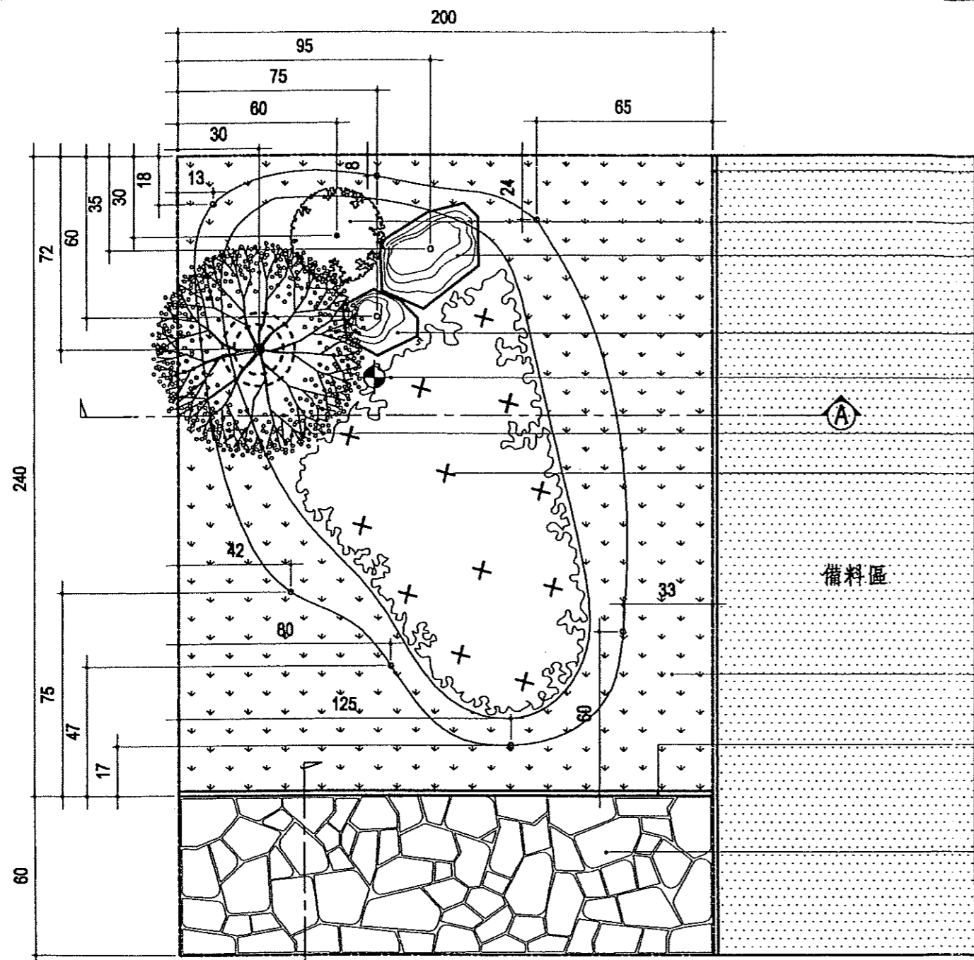
平面圖 S=1/20
