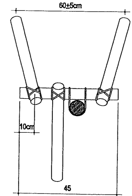
支柱上視示意圖 S=1/10
