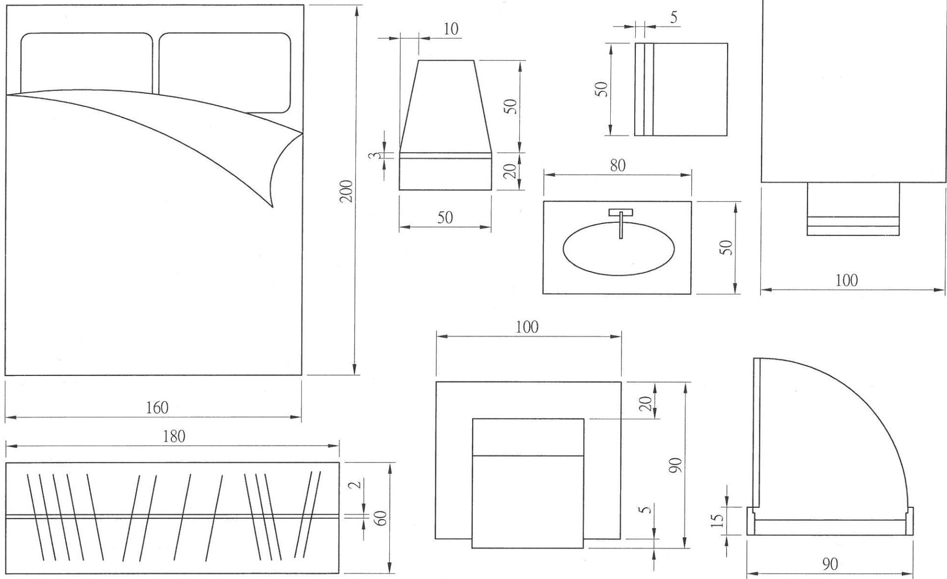
圖名 傢俱繪製 比例 1:20 單位 公分 室一仁 座號 姓名
